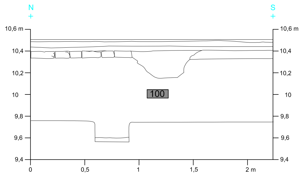
ALÇAT MUR N - S
