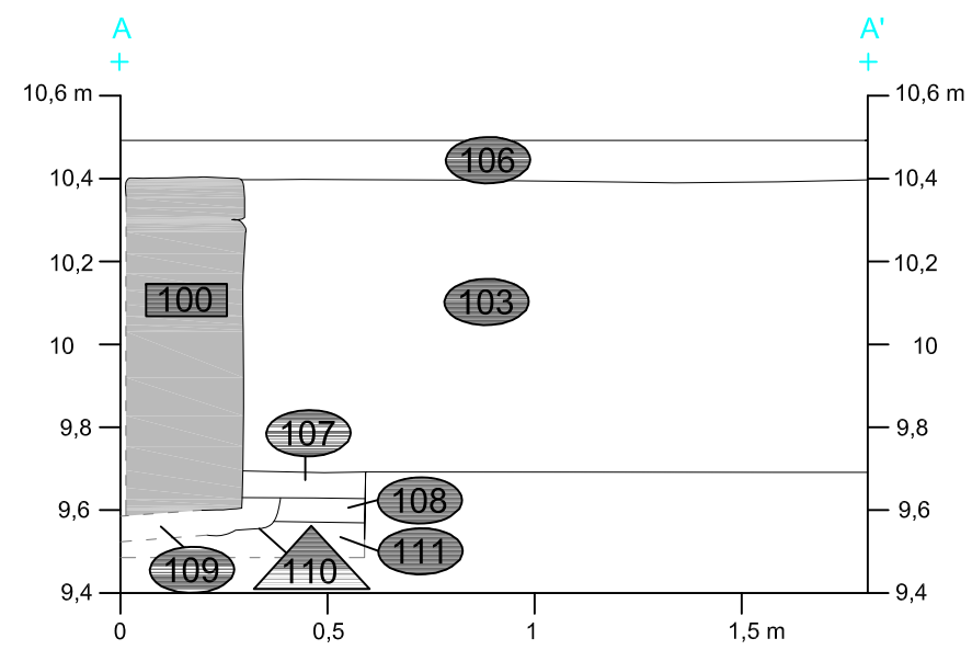
SECCIÓ A - A'
