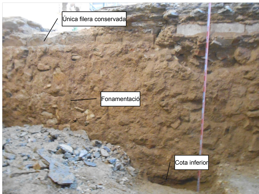
Foto 6 Alçat total conservat del mur UE 100
